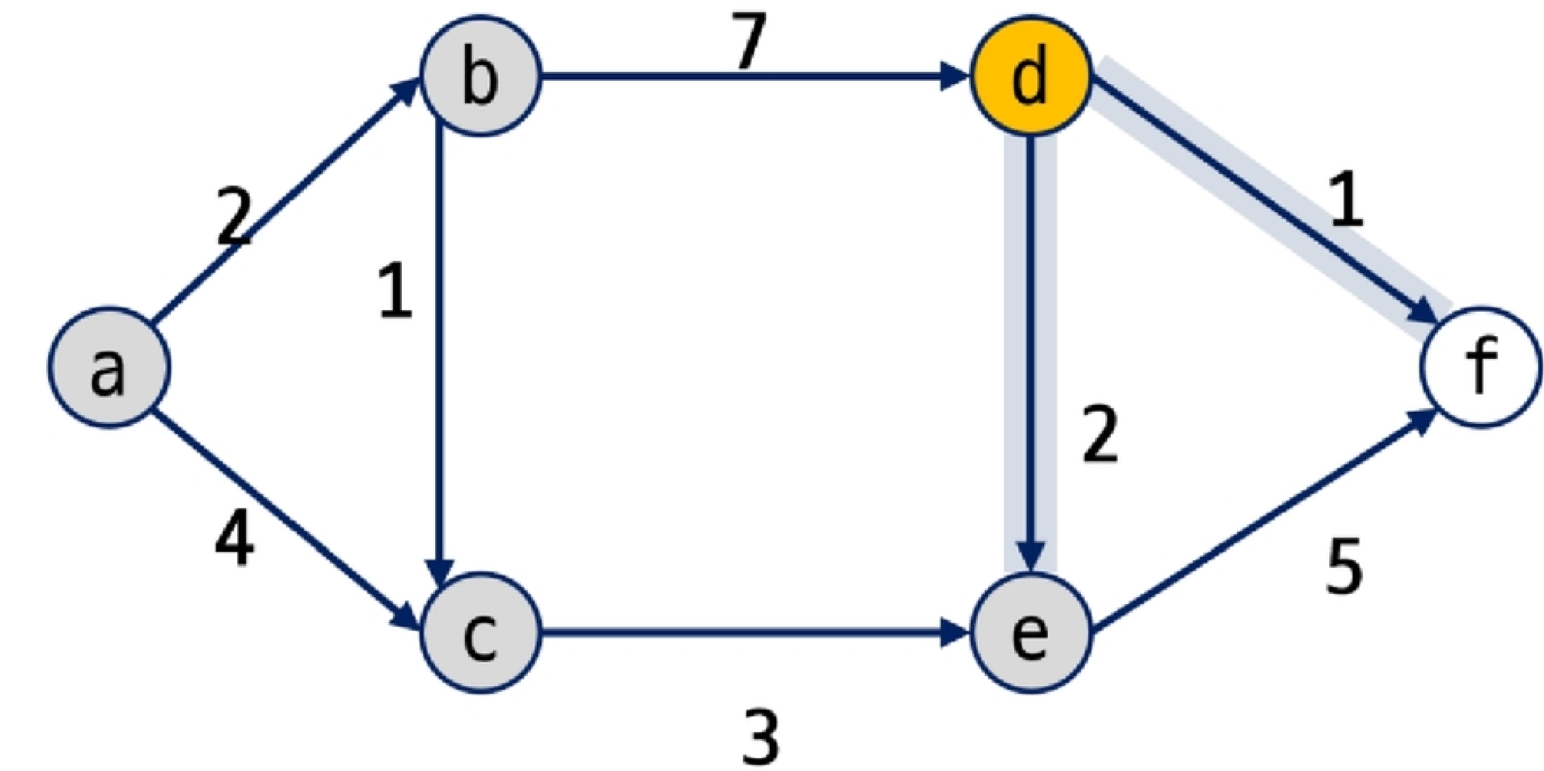
<그림26_SW문제해결 응용_그래프의 최소비용 문제_Dijkstra 알고리즘13>
