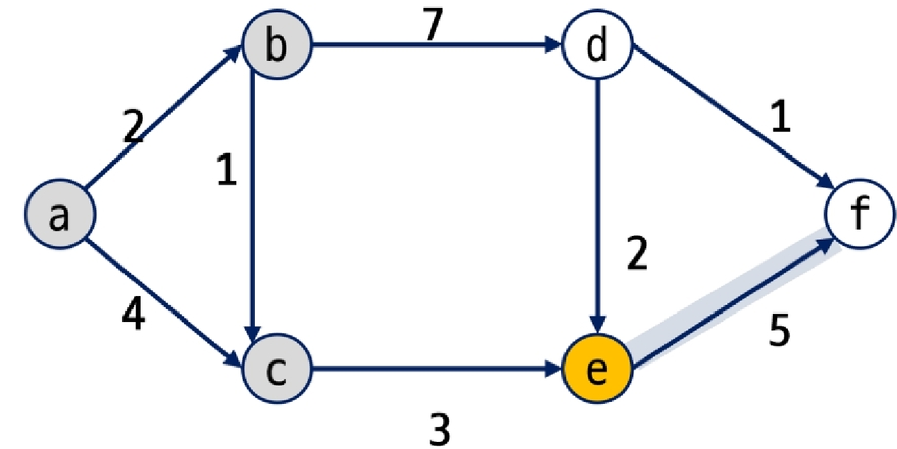
<그림24_SW문제해결 응용_그래프의 최소비용 문제_Dijkstra 알고리즘11>
