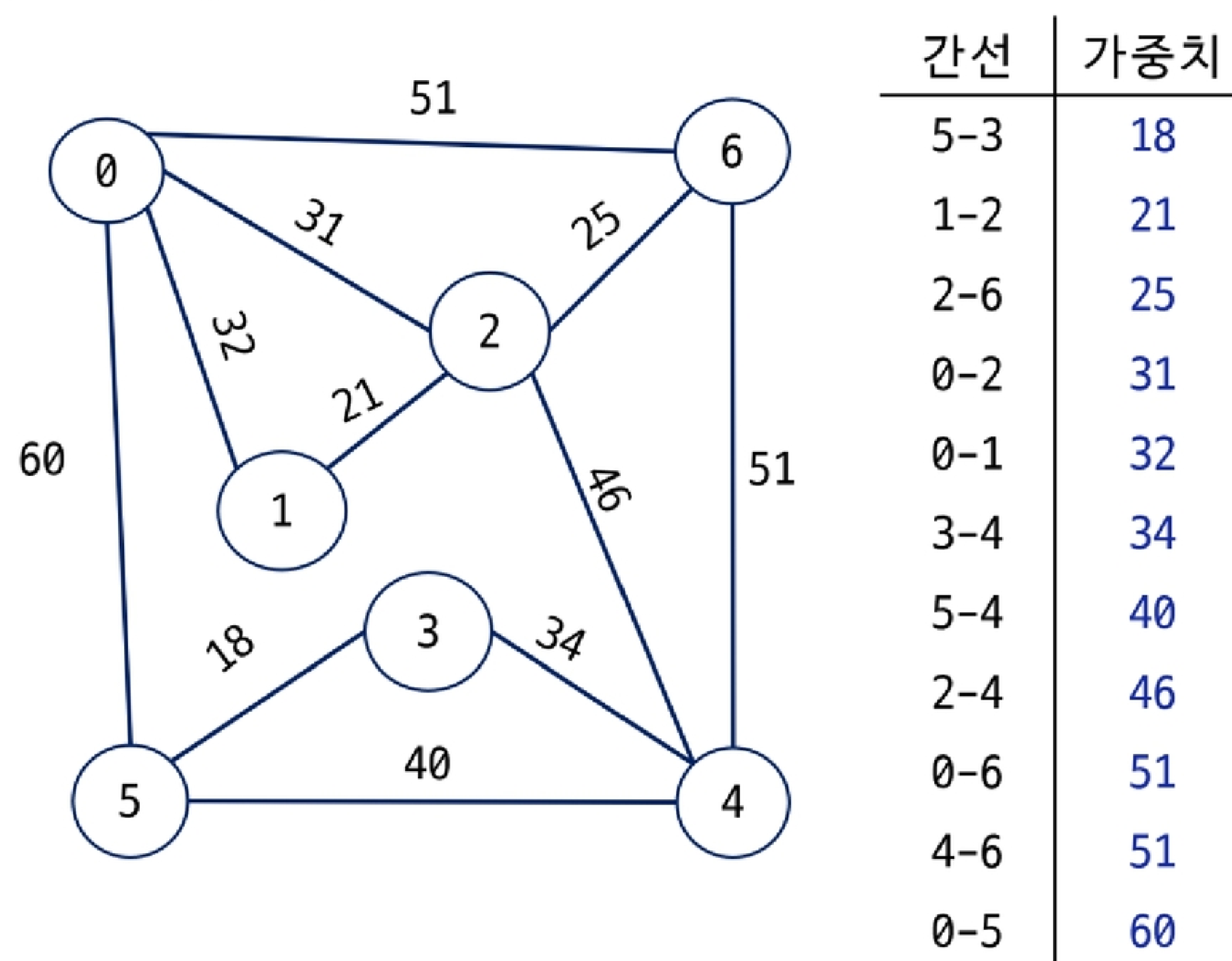
<그림10_SW문제해결 응용_그래프의 최소비용 문제_Kruskal 알고리즘>
