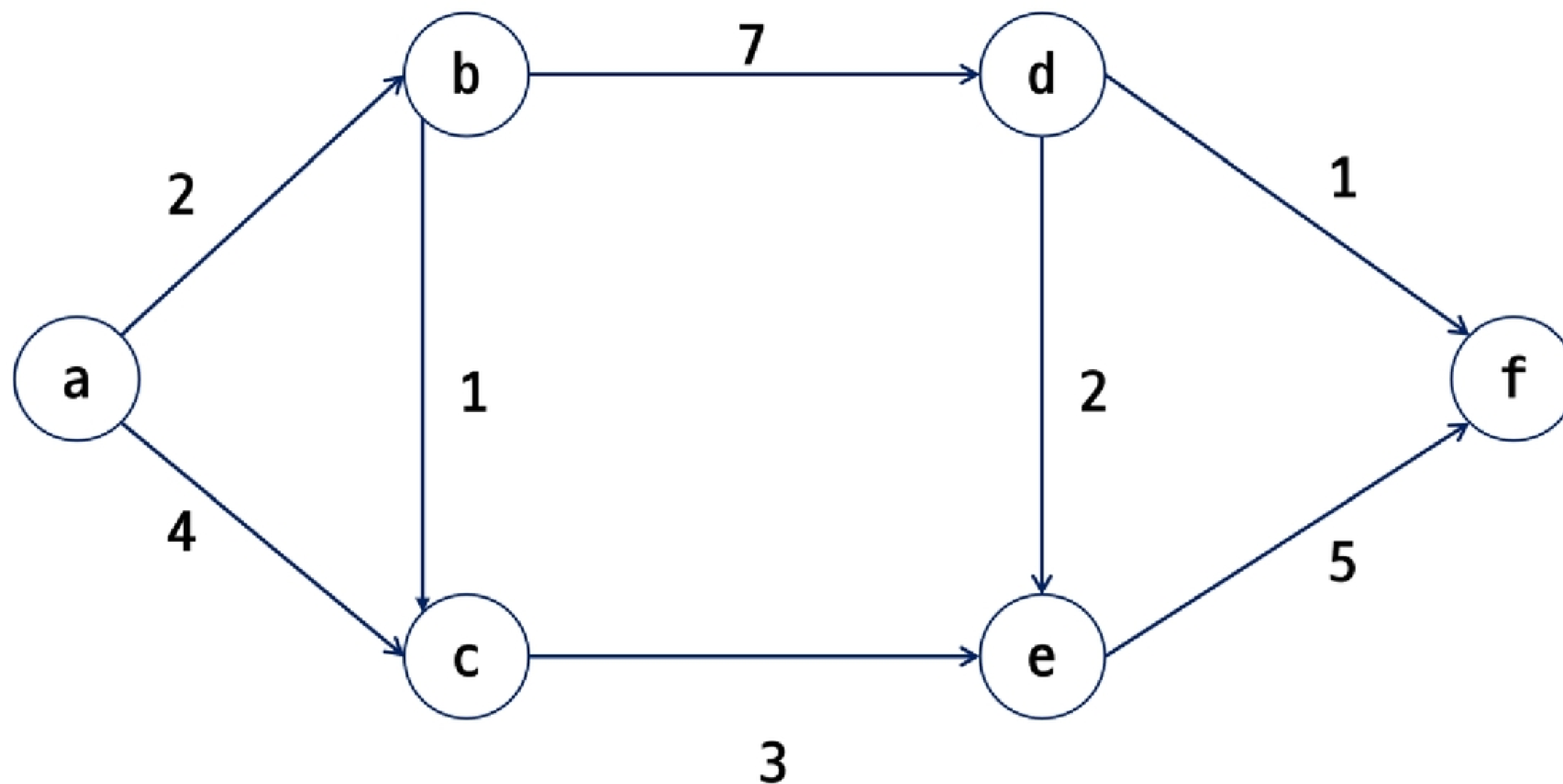
<그림14_SW문제해결 응용_그래프의 최소비용 문제_Dijkstra 알고리즘1>
