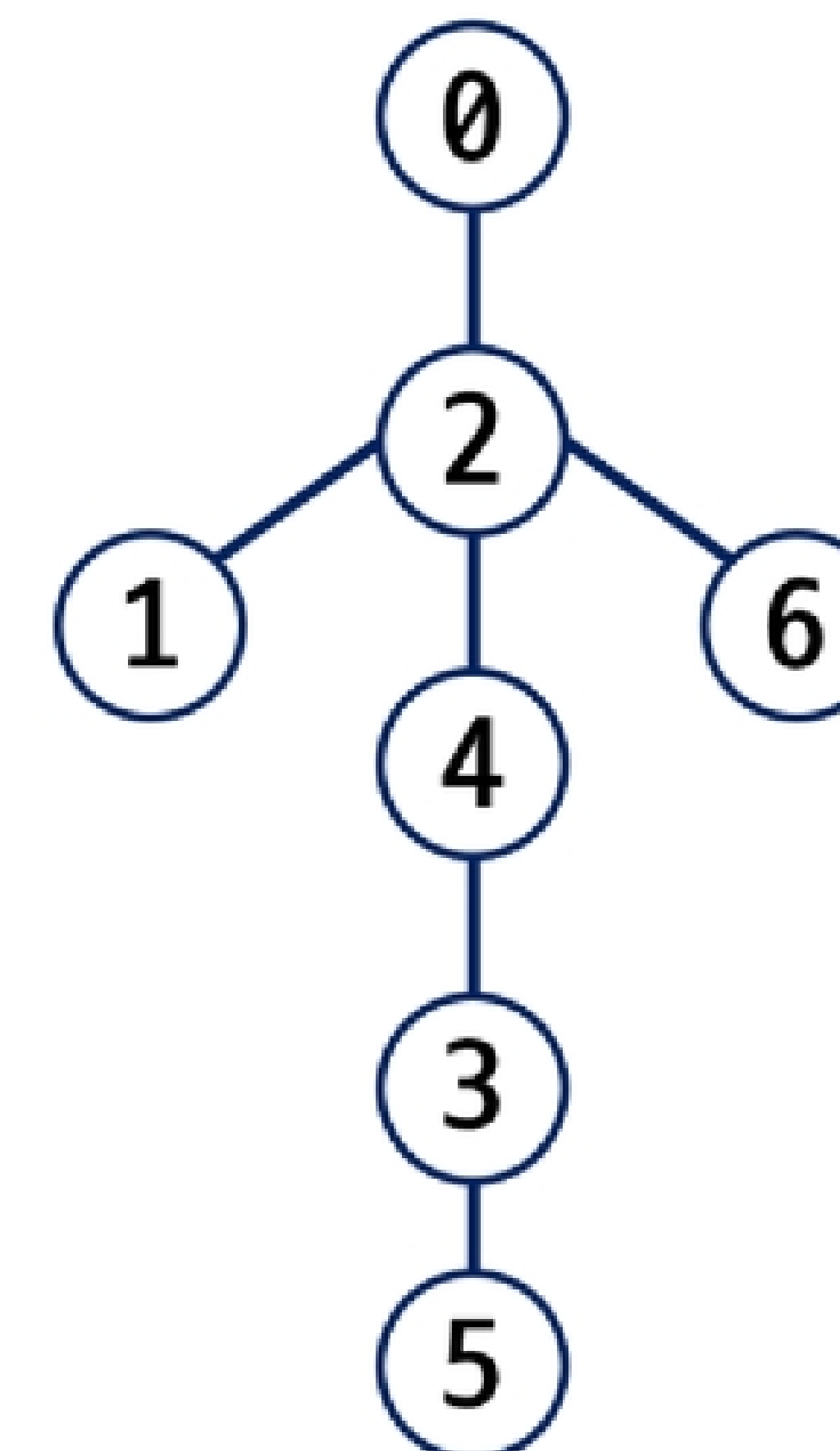
〈그림6_SW문제해결 응용_그래프의 최소비용 문제_MST 표현6〉
