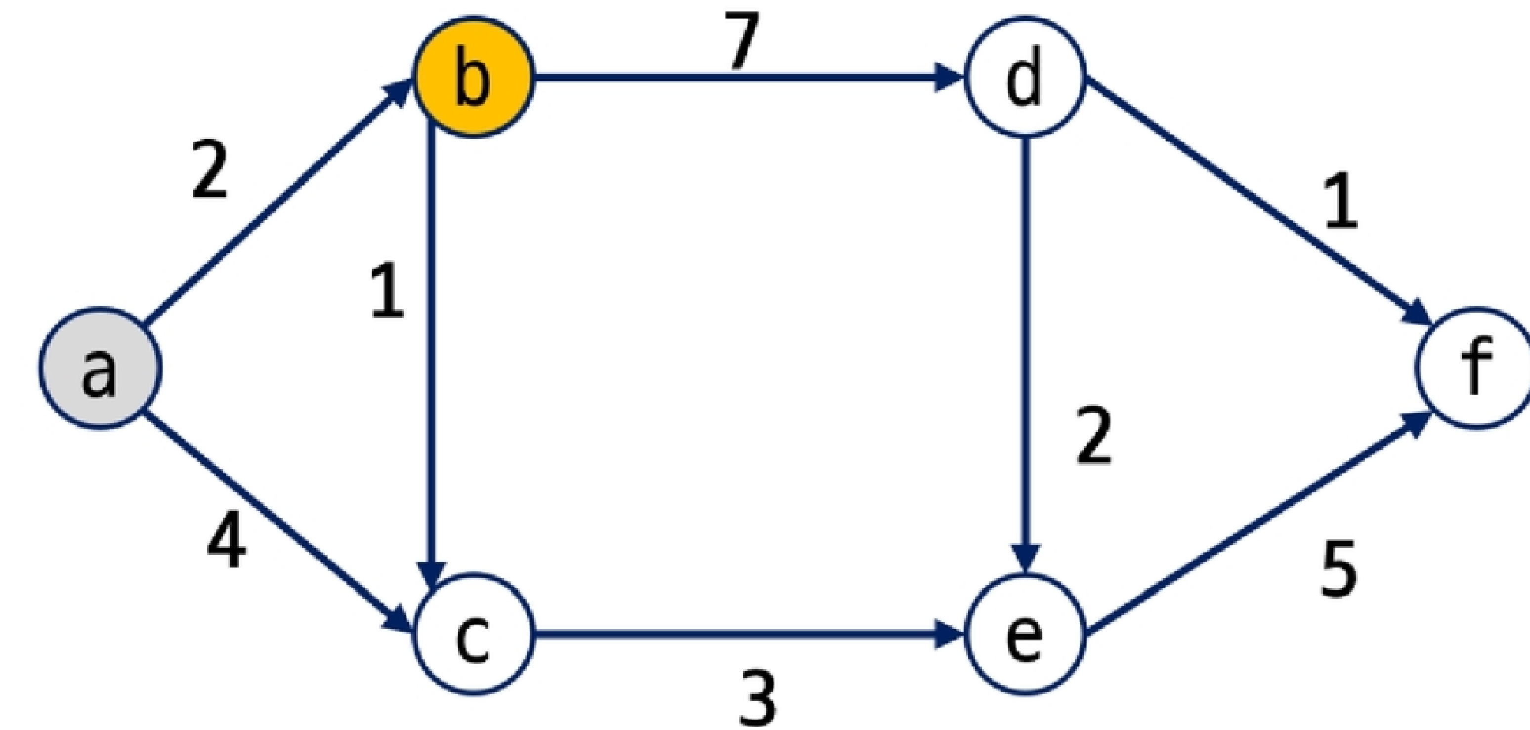
<그림18_SW문제해결 응용_그래프의 최소비용 문제_Dijkstra 알고리즘5>
