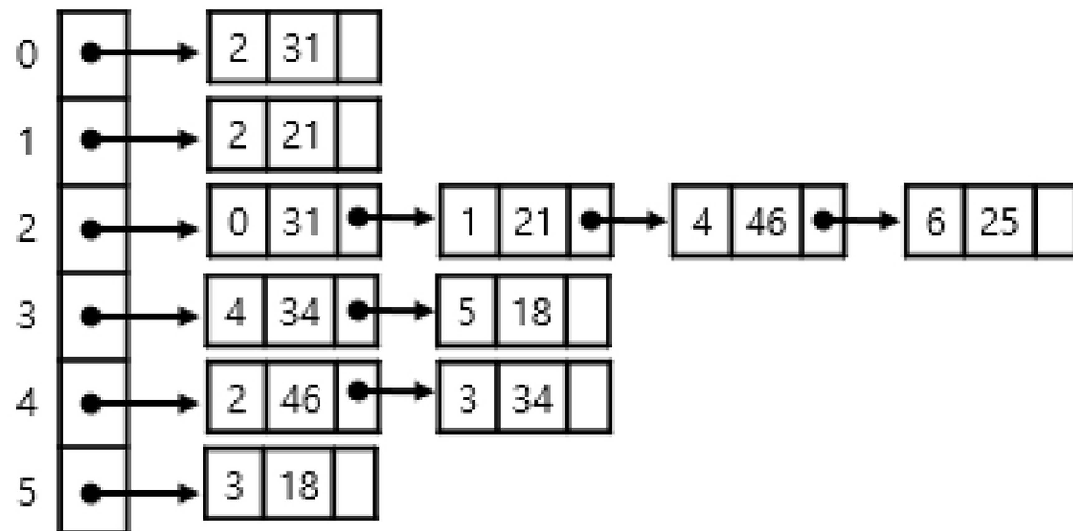
〈그림5_SW문제해결 응용_그래프의 최소비용 문제_MST 표현5〉
