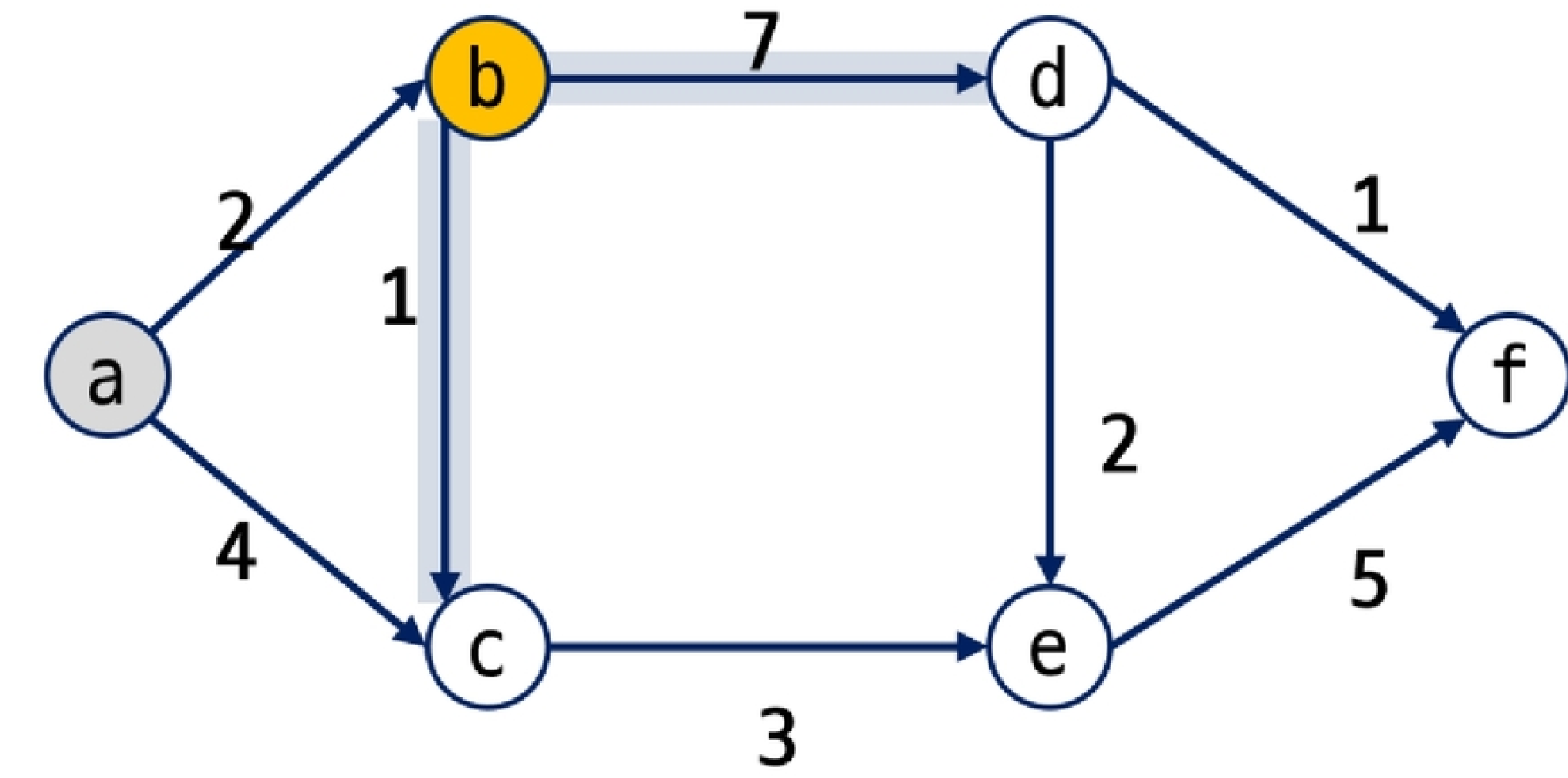
<그림20_SW문제해결 응용_그래프의 최소비용 문제_Dijkstra 알고리즘>
