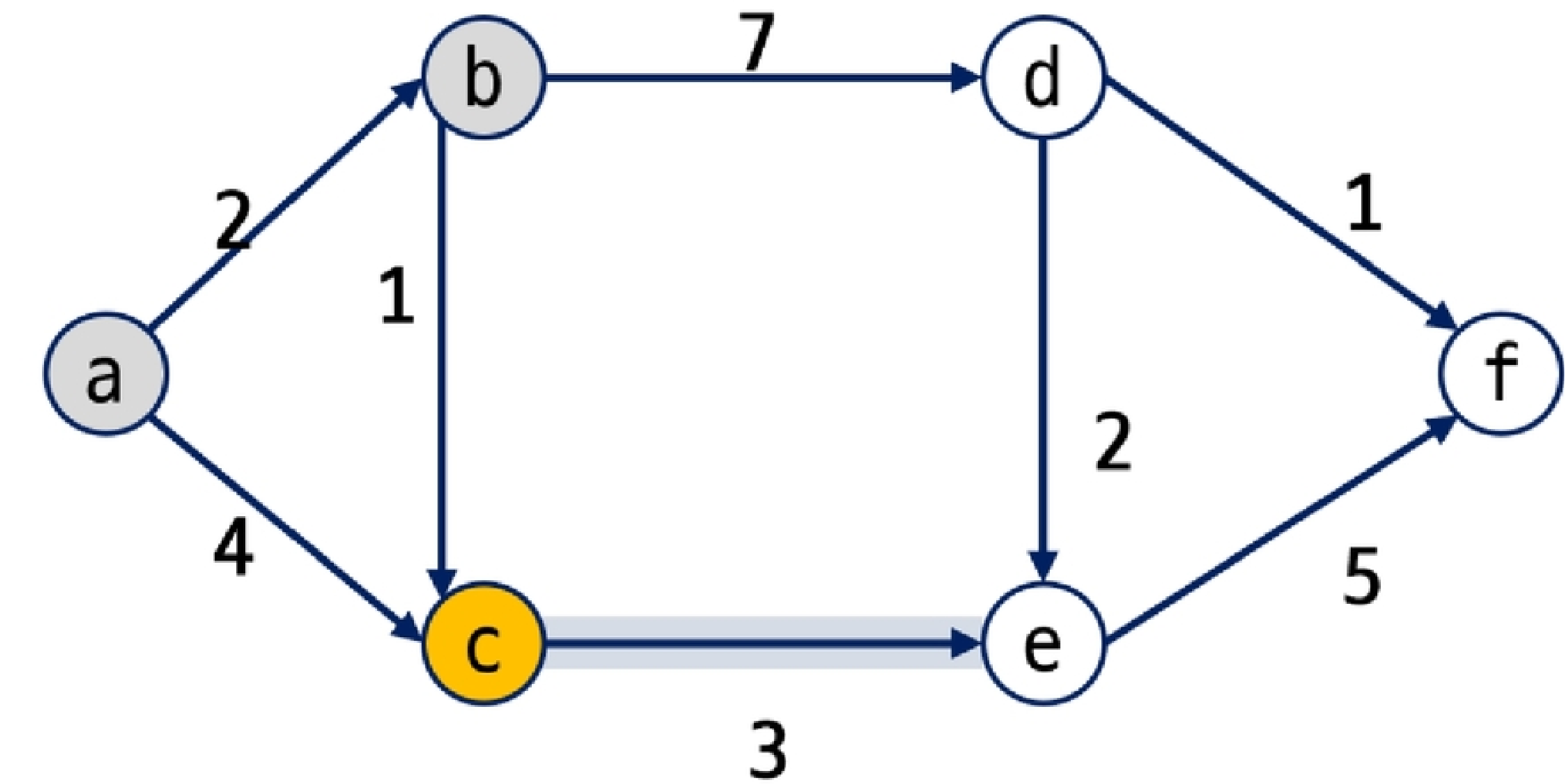
<그림22_SW문제해결 응용_그래프의 최소비용 문제_Dijkstra 알고리즘9>
