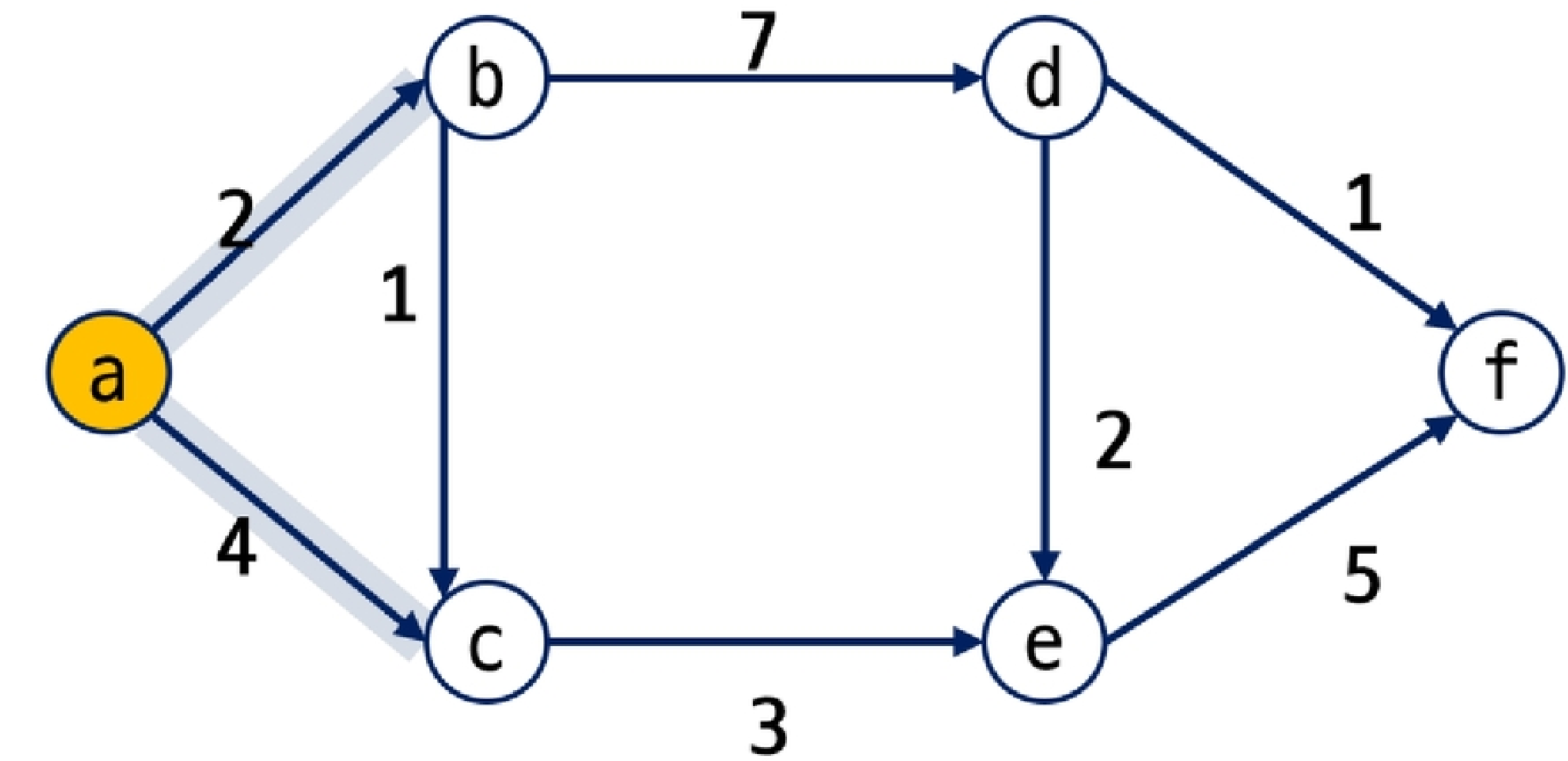
<그림16_SW문제해결 응용_그래프의 최소비용 문제_Dijkstra 알고리즘3>
