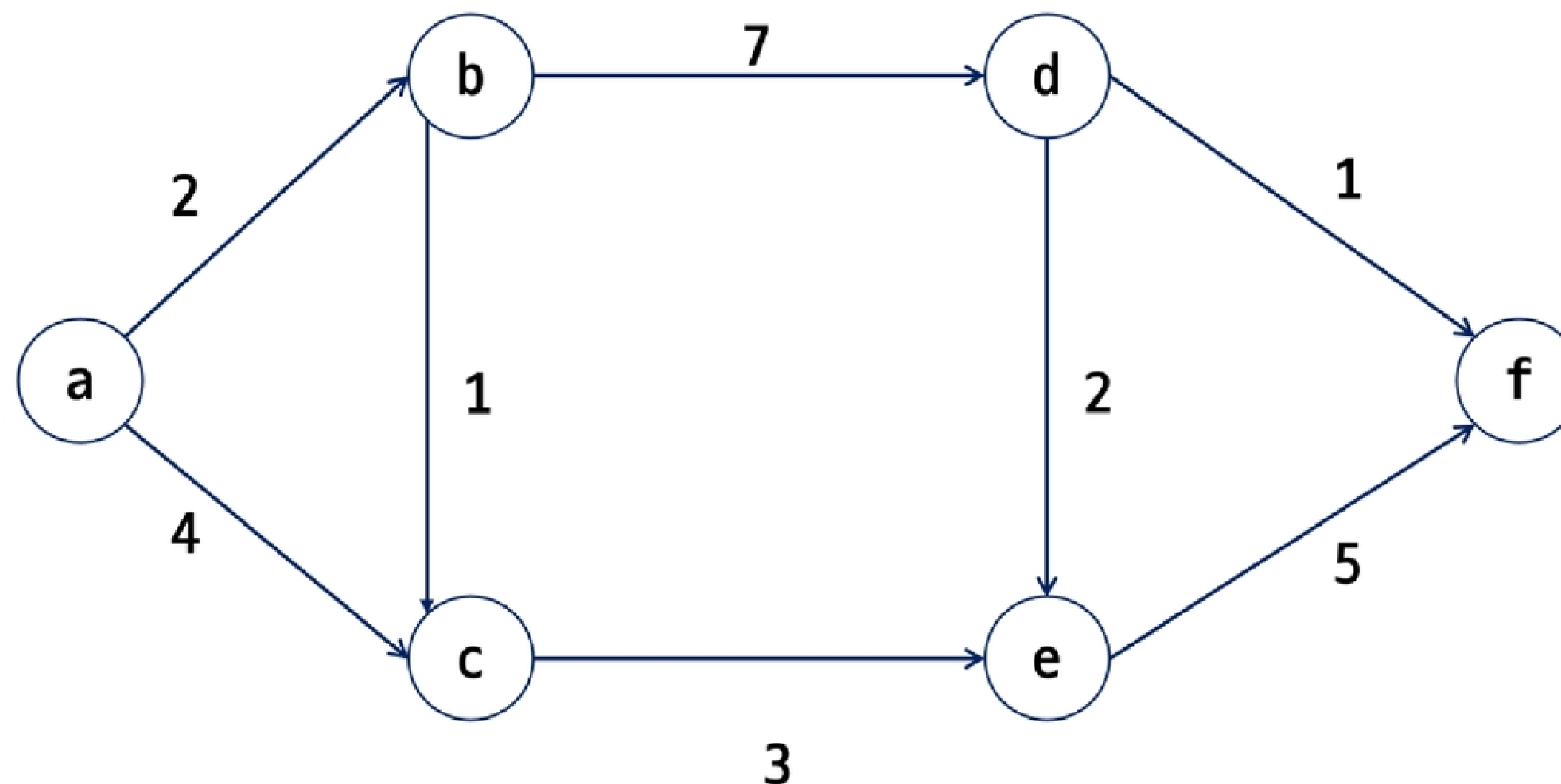
<그림14_SW문제해결 응용_그래프의 최소비용 문제_Dijkstra 알고리즘1>
