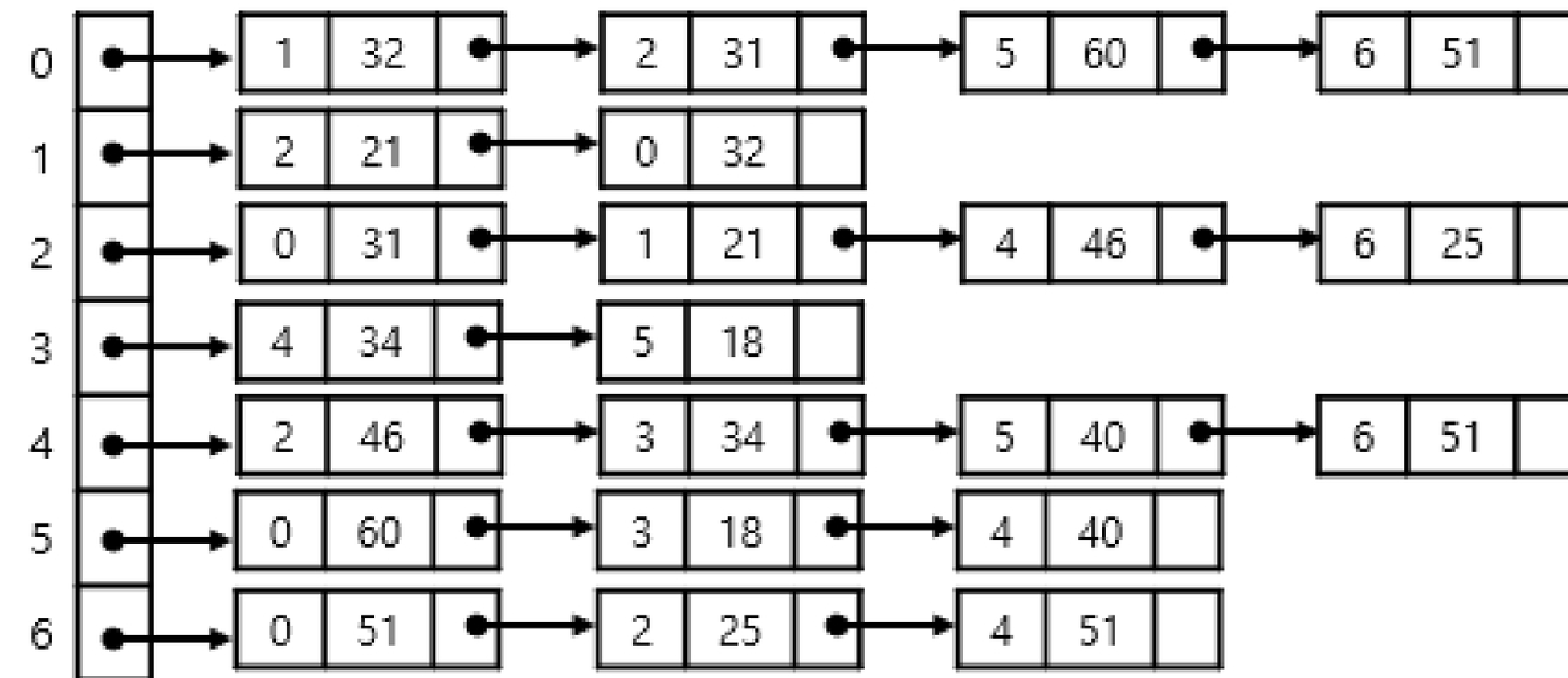
<그림3_SW문제해결 응용_그래프의 최소비용 문제_가중치 인접리스트>
