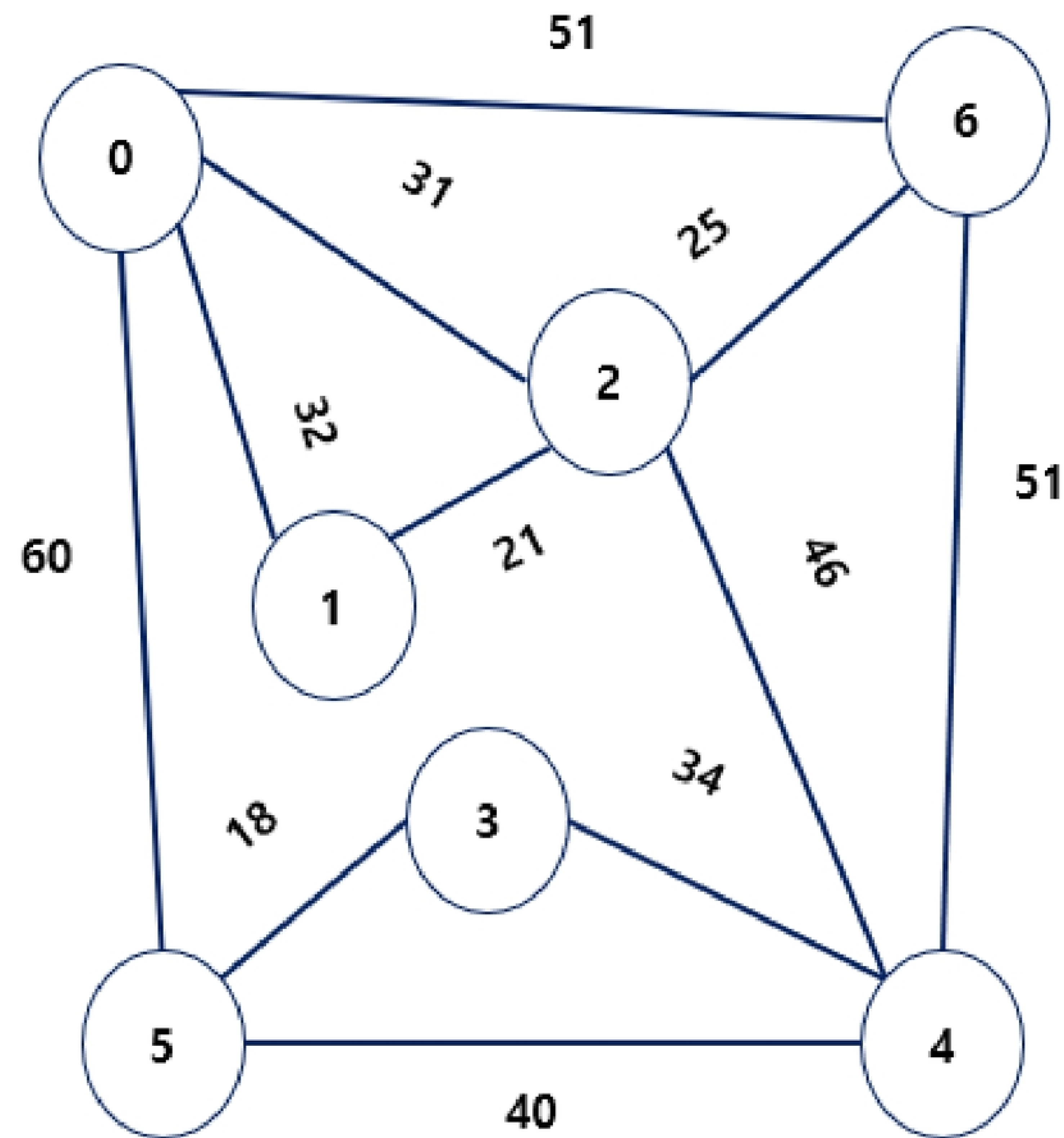
<그림9_SW문제해결 응용_그래프의 최소비용 문제_Prim 알고리즘3>
