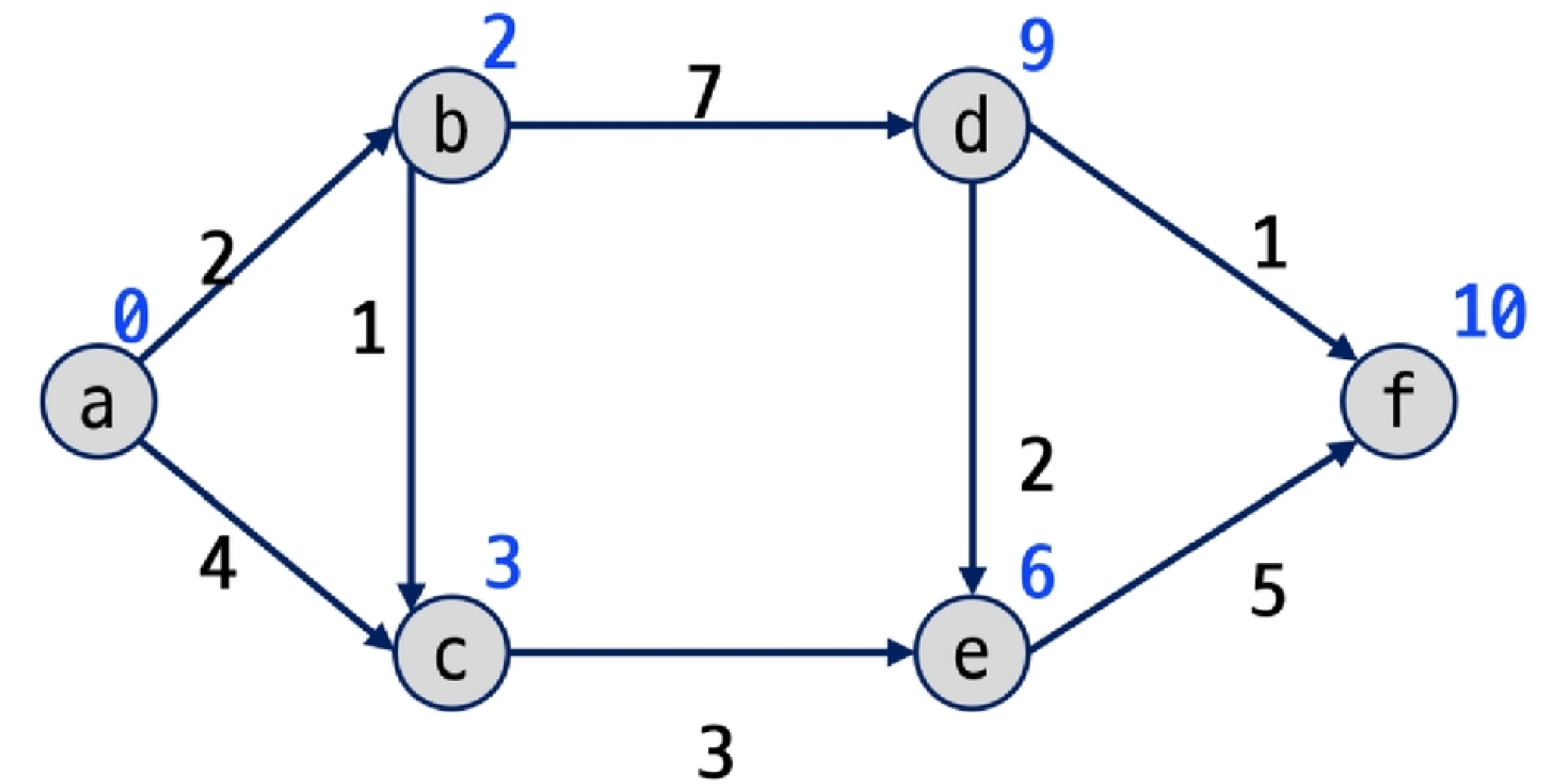
<그림30_SW문제해결 응용_그래프의 최소비용 문제_Dijkstra 알고리즘17>
