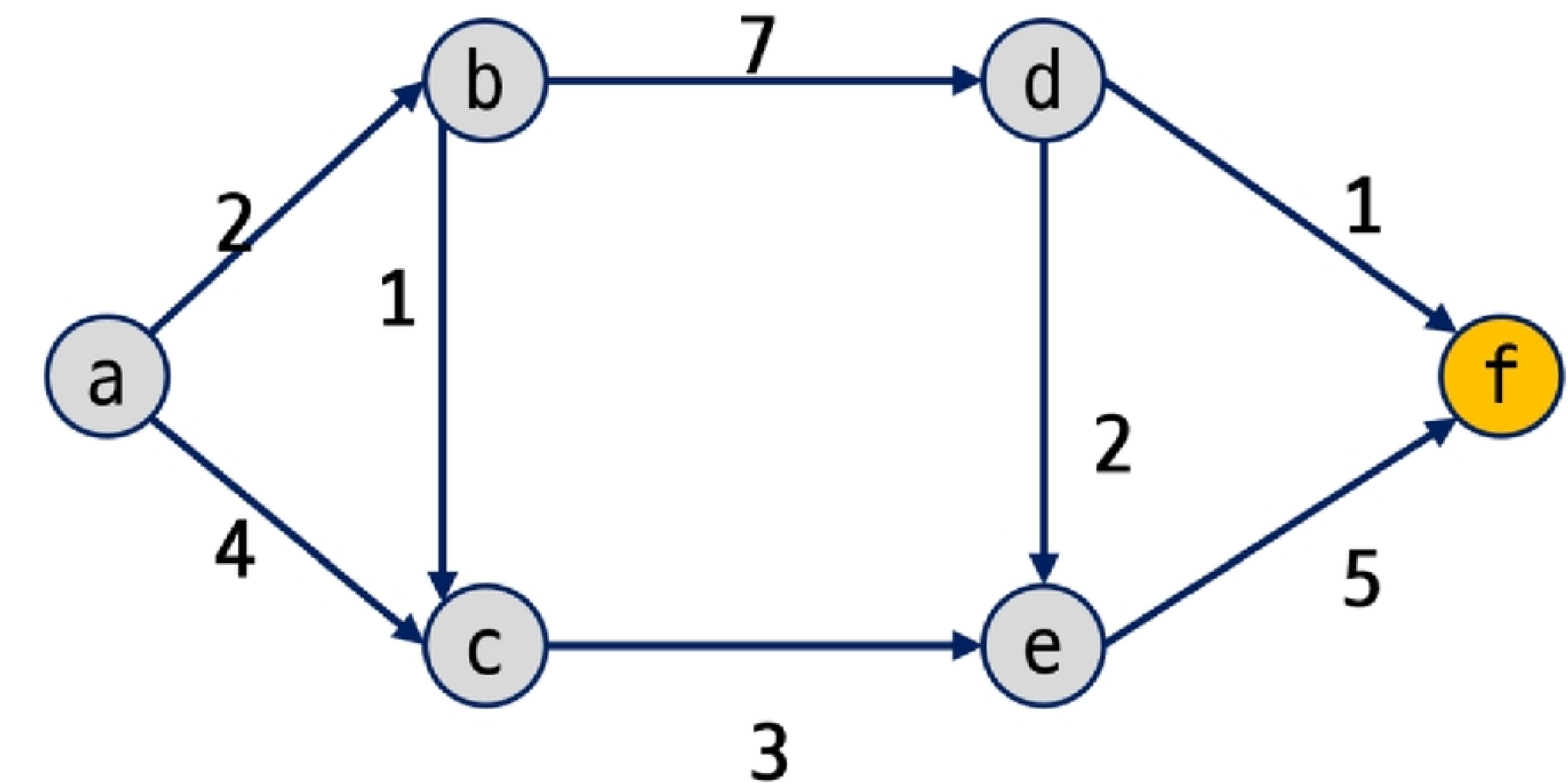
<그림28_SW문제해결 응용_그래프의 최소비용 문제_Dijkstra 알고리즘15>
