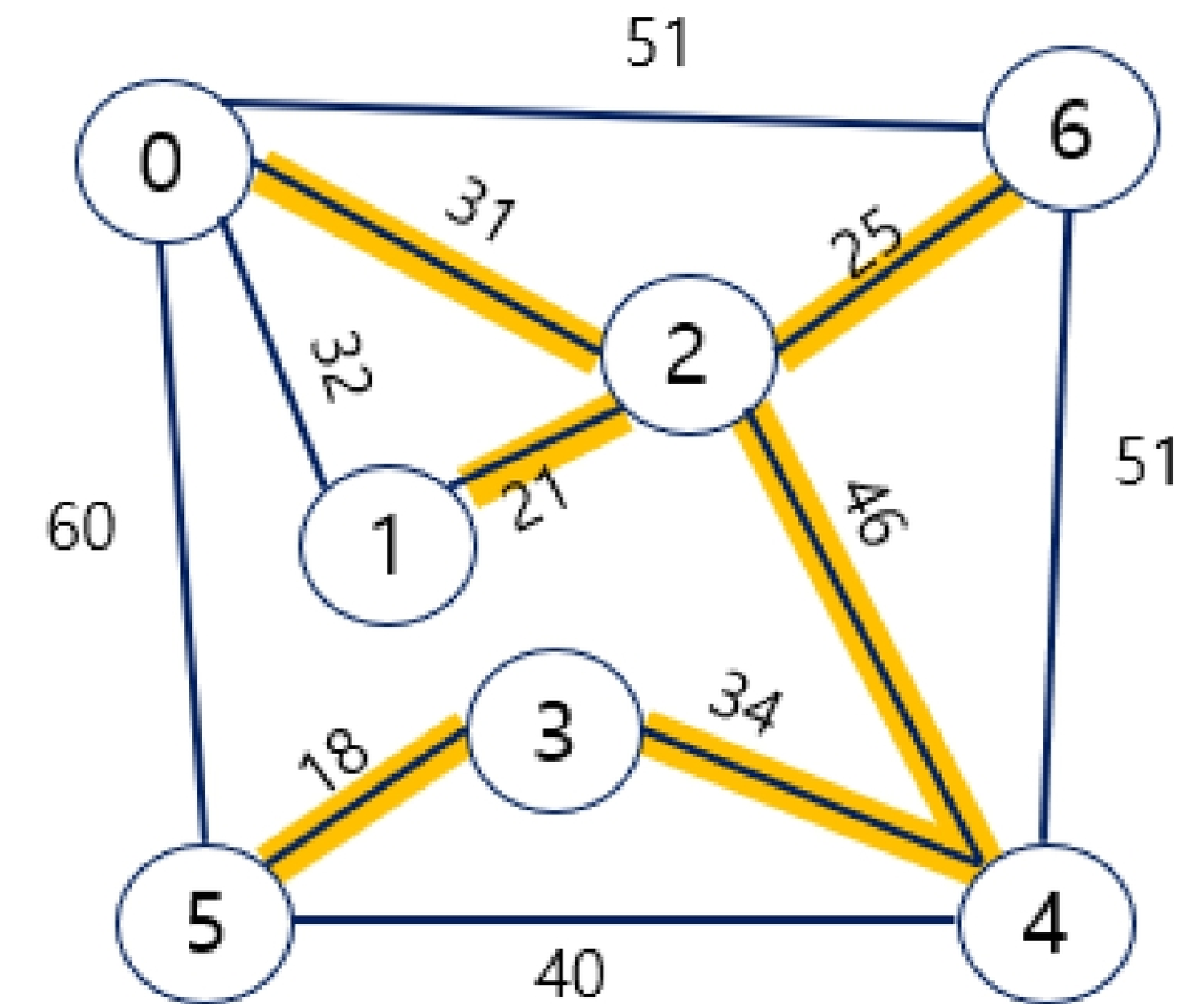
<그림1_SW문제해결 응용_그래프의 최소비용 문제_그래프에서의 MST>
